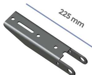
FR0014B DOBRADIÇA DO TOMBADOR INFERIOR ECOPLATÉ (ZINCADO BRANCO)
