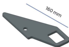
FE0020A ENGATE FÊMEA INFERIOR
