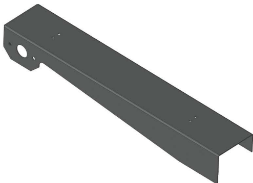
FD0251 SUPOORTE LANTERNA DIANTEIRO DOLLY RODOFORT LADO DIREITO
