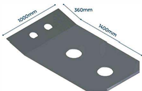
FR0600 MESA PINO REI DA CARRETA RANDON CHAPA 7,94mm
