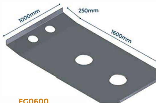
FG0600A MESA PINO REI DA CARRETA GUERRA CHAPA 9,54mm
