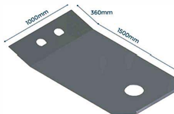
FR0601 MESA PINO REI 1º BITREM RANDON CHAPA 7,94mm
