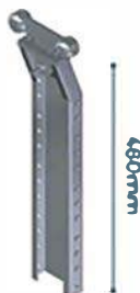
FRP0803A - PRETO EPÓXI FRZ0803A - ZINCADA CABEÇA DA COLUNA MÓVEL SIDER RANDON MOD. 2
