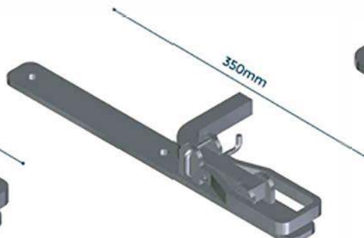
F4076C DOBRADIÇA TRUCK DIANTEIRA LADO DIREITO F4076D DOBRADIÇA TRUCK DIANTEIRA LADO ESQUERDO
