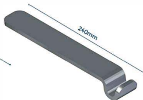
F4076 GANCHO PARA DOBRADIÇA DO TRUCK
