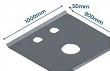
FR0602 MESA PINO REI 2º BITREM RANDON CHAPA 7,94mm
