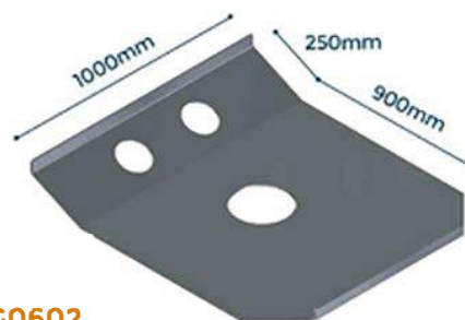
FG0602 MESA PINO REI 2º BITREM GUERRA CHAPA 7,94mm
