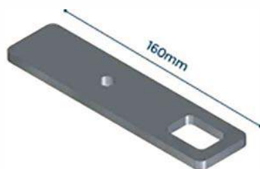
FG0018 ENGATE FÊMEA DA GRADE TRASEIRA
