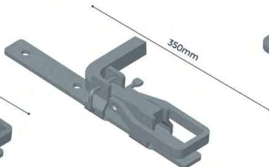
F4076C DOBRADIÇA TRUCK DIANTEIRA LADO DIREITO
