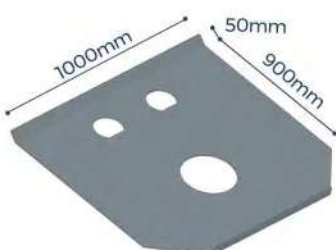
FR0602 MESA PINO REI 2º BITREM RANDON CHAPA 7,94mm
