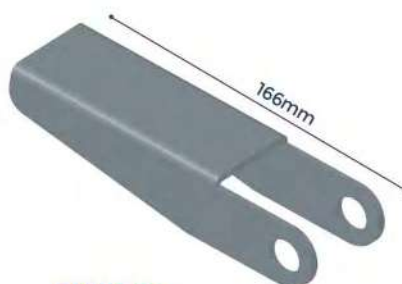
FN0014 DOBRADIÇA DO TOMBADOR INFERIOR
