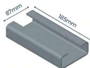
FN0122 ENCAIXE DO FUEIRO
