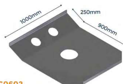
FG0602 MESA PINO REI 2º BITREM GUERRA CHAPA 7,94mm
