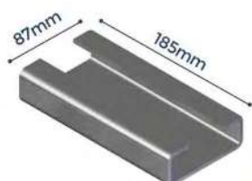
FL0122 ENCAIXE DO FUEIRO
