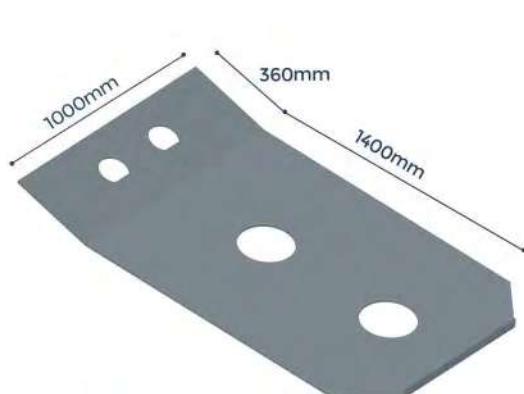
FR0600 MESA PINO REI DA CARRETA RANDON CHAPA 7,94mm
