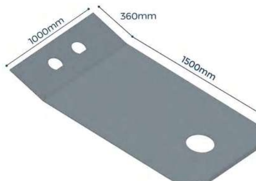
FR0601 MESA PINO REI 1º BITREM RANDON CHAPA 7,94mm
