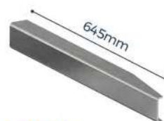
F4170E REFORÇO DAS EXTREMIDADES DA LÂMINA (CH. 4,75mm)
