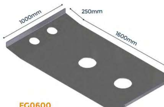
FG0600 MESA PINO REI DA CARRETA GUERRA CHAPA 7,94mm
