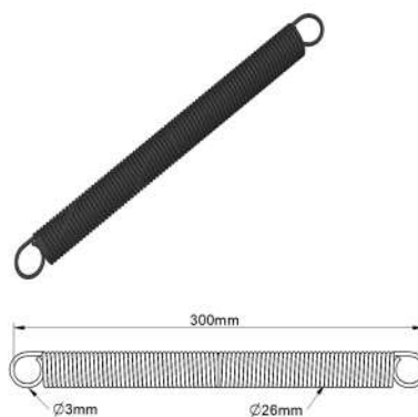
Mola do Para-Choque 300mm
