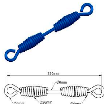
Mola Patim de Freio Longa Dupla do Scania 210mm
