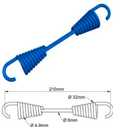
Mola Patim de Freio Dupla Móvel 134 Gancho Curto 210mm
