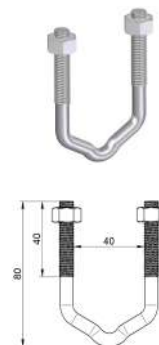
PRESILHA "W" DA TAMPA com porcas (40mm interna) Embalagens com 50 unidades F4027A
