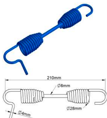
Mola Patim de Freio Dupla Móvel com Gancho Longo 210mm
