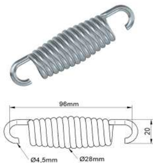
Mola Patim de Freio Sc 110/111/F112/ F113/K112/K113/L75/L76/Lk140/ Lk141/R112/R113/R142/R143/T112/ T113/T142
