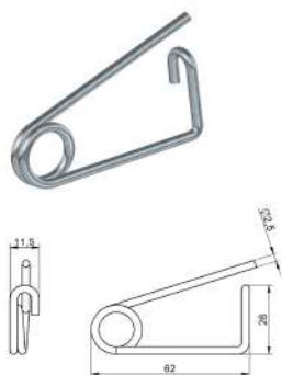
Joaninha Pequena (2,5X62mm) F4054B - zincado branco
