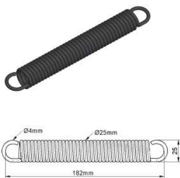
Mola do Para-Choque Guerra 190mm
