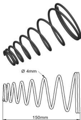
Mola Retorno Cuica Freio Central Conica Tipo 16" Master
