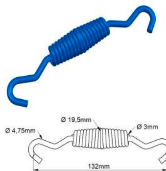
Mola Siri Patim de Freio Retenção Dianteiro/Traseiro Master Gancho Móvel Sistema Bendix/Master
