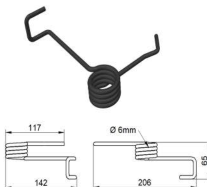
Mola Para Tranca da Basculante Lado Esquerdo (F4114G)
