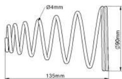
Mola Camera de Serviço e Spring Brake 20
