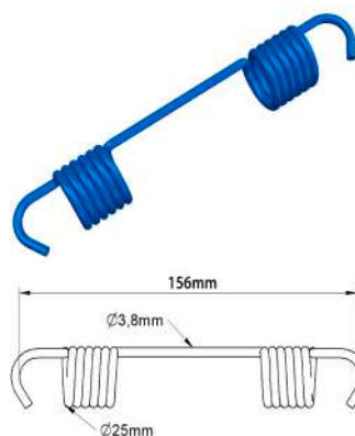
Mola Patim Freio Retorno Dianteiro/Traseiro 165mm - Mbb 710 Lo712 812 Vwc 8120 8150E 9150E Worker 8140 8150 Delivery Ford 815E Agrale 9200 Volare A8 W8 W9
