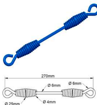
Mola Patim de Freio Longa Dupla do Scania 114/124 - 270mm
