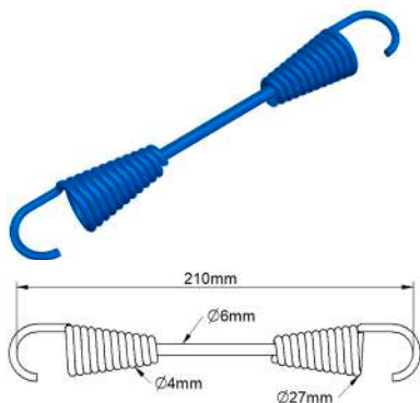
Mola Patim de Freio Carreta Rodoviária Dupla Móvel 210mm
