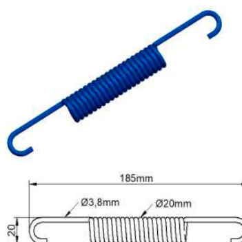
Mola Patim de Freio Inferior Vwc
