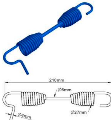
Mola Patim de Freio Bendix Dupla Móvel com 1 Gancho Longo 210mm
