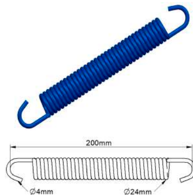
Mola Reta Patim Freio Trucks e Carretas Cód. Original: 211300010 FM0022 - cor azul FM0022A - sem pintura
