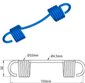
Mola de Tração Patim de Freio Mb Caminhão Mbb Accelo 815 e Ônibus Lo815 E Lo916 Caminhão Ford C1118
