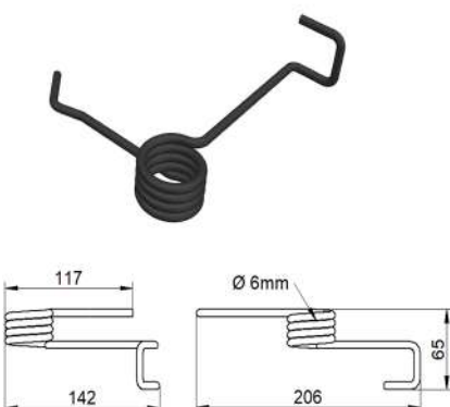
Mola Para Tranca da Basculante Lado Direito (F4114H)
