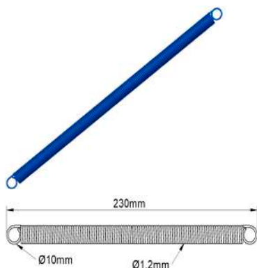
Mola do Acelerador 230mm Mb FM0019 - cor azul FM0019A - sem pintura
