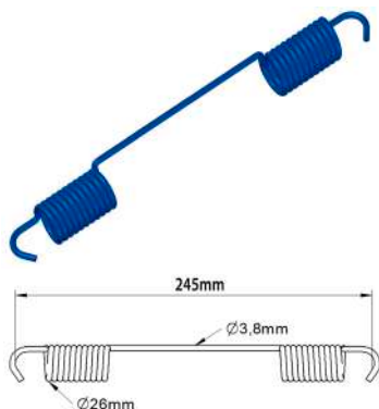
Mola Patim Freio Dianteiro/Traseiro Mbb 1313 1513 1516 1517 1518 1620 1720 Todos Freio a Ar 253mm
