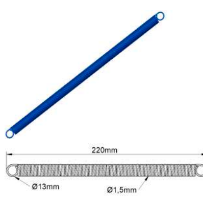
Mola do Acelerador 220mm Mb FM0020 - cor azul FM0020A - sem pintura
