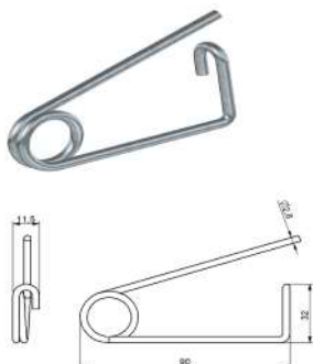
Joaninha (2,8X90mm) F4054 - zincado branco
