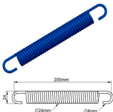
Mola Patim Freio Carreta Randon FM0016 - cor azul FM0016A - sem pintura
