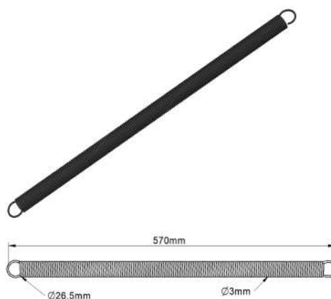
Mola do Para-Choque 570mm
