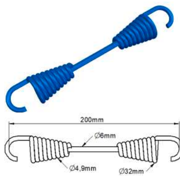
Mola Patim de Freio Carreta Sistema Master Dupla Móvel 200mm
