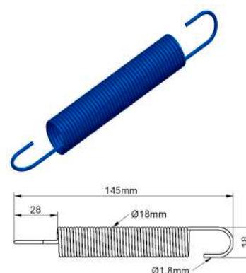
Mola Freio Motor Mb FM0018 - cor azul FM0018A - sem pintura
